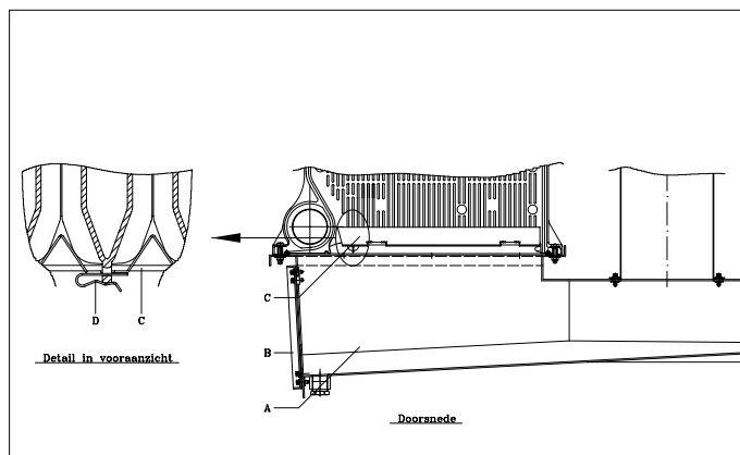
Afb. 19 Doorsnedetekening
