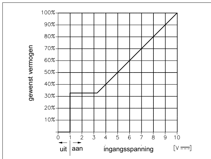
Afb. 10 Externe ketelbesturing d.m.v. analoog (0-10 V) signaal
