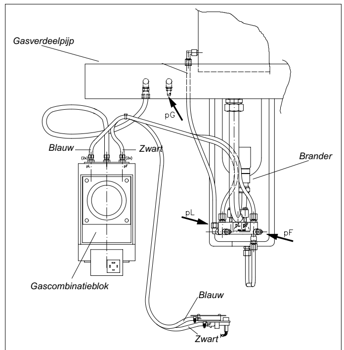
Afb. 16 Drukverschil meetpunten
