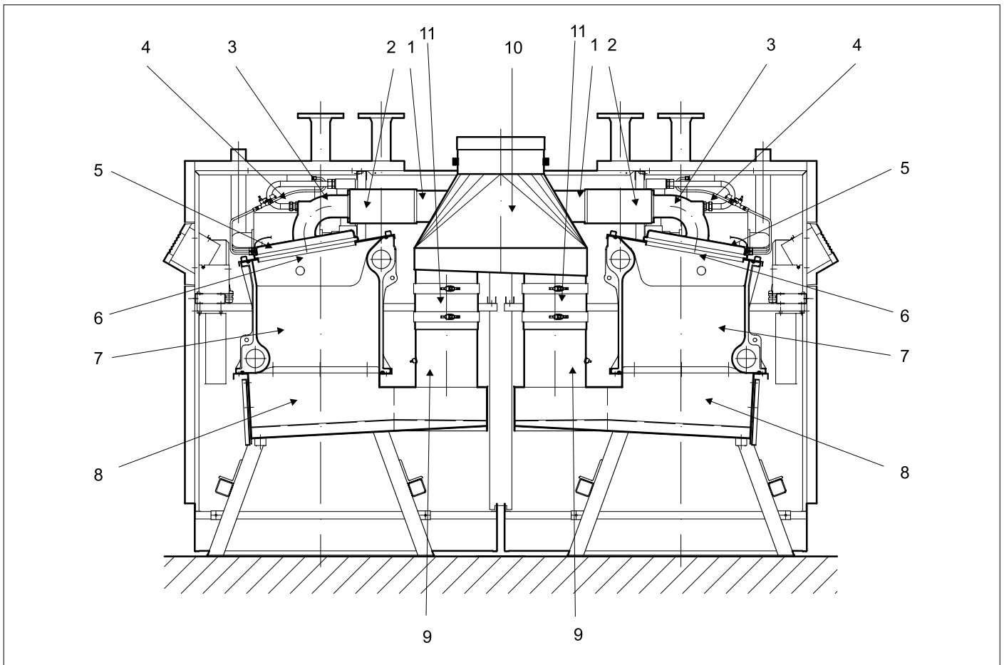
Afb. 07 Doorsnede rechterzijaanzicht
