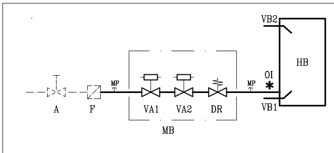
Afb. 12 Schematische uitvoering gasapparatuur
