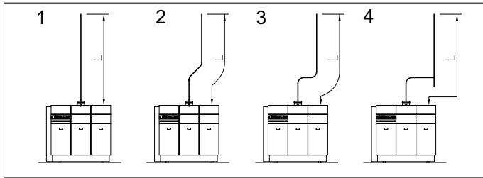
Afb. 04 Uitvoering rookgasafvoerleiding
