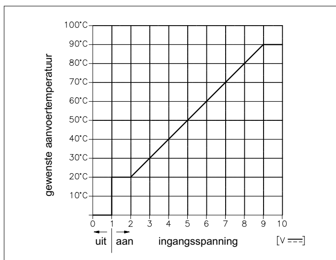
Afb. 09 Interne ketelbesturing d.m.v. analoog (0-10 V) signaal (standaardinstelling)
