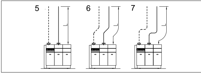
Afb. 05 Uitvoering luchttoe- en rookgasafvoer
