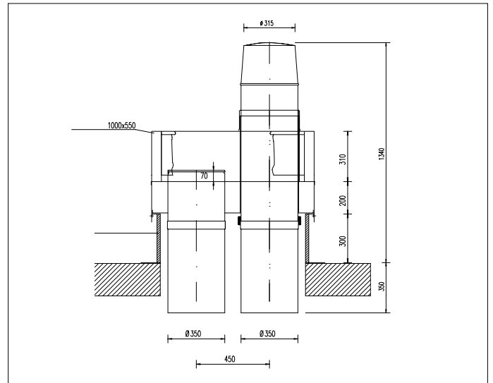
Afb. 06 Remeha dakdoorvoer tbv Gas 6002 (ECO) Ketels
