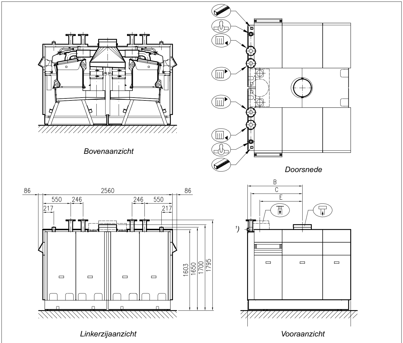
Afb. 01 Aanzichttekeningen
