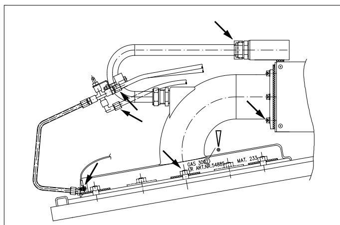
Afb. 18 Bevestigingspunten branderunit
