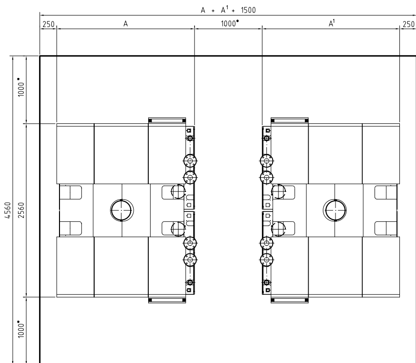
Afb. 02 Opstellingsmogelijkheden in het ketelhuis
